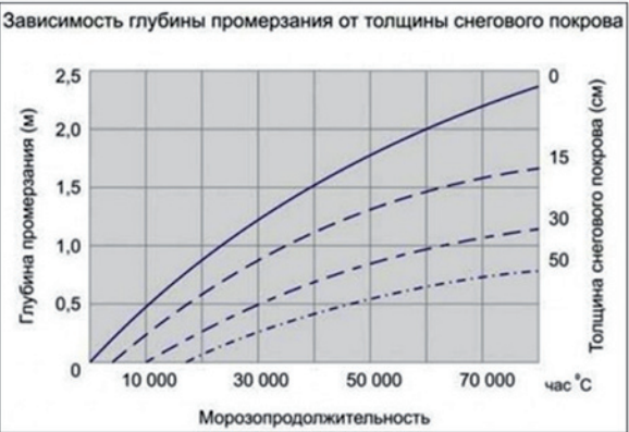
Рисунок 10. График зависимости промерзания грунта в России
