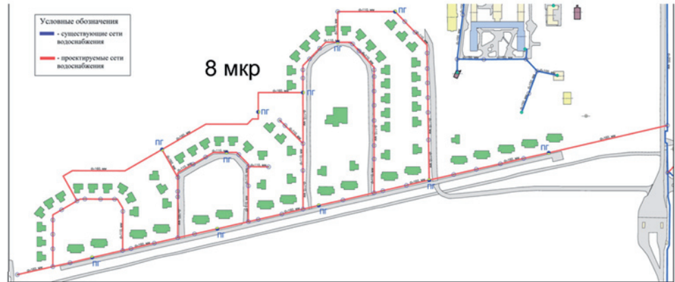
Рисунок 22. Схема размещения объектов водоснабжения микрорайона № 8
