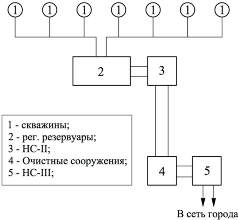
Рисунок 17. Технологическая схема проектируемого подземного водозабора
