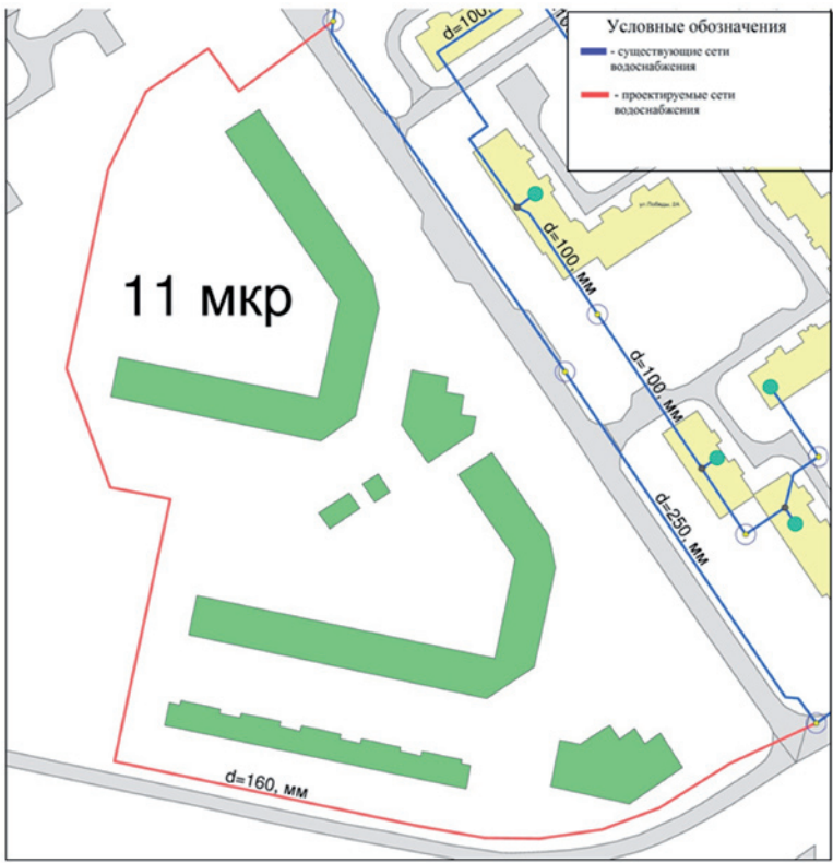
Рисунок 21. Схема расположения объектов водоснабжения микрорайона № 11
