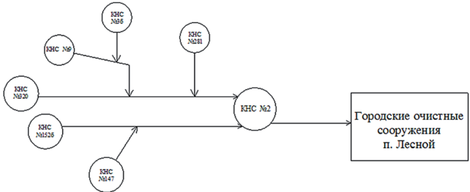
Рис. 4 Принципиальная схема передачи стоков по технологической зоне водоотведения ФГУП «Комбинат «Электрохимприбор»
