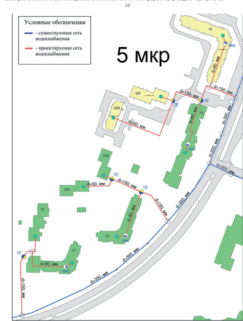
Рисунок 18. Схема расположения объектов водоснабжения южной части микрорайона № 5
