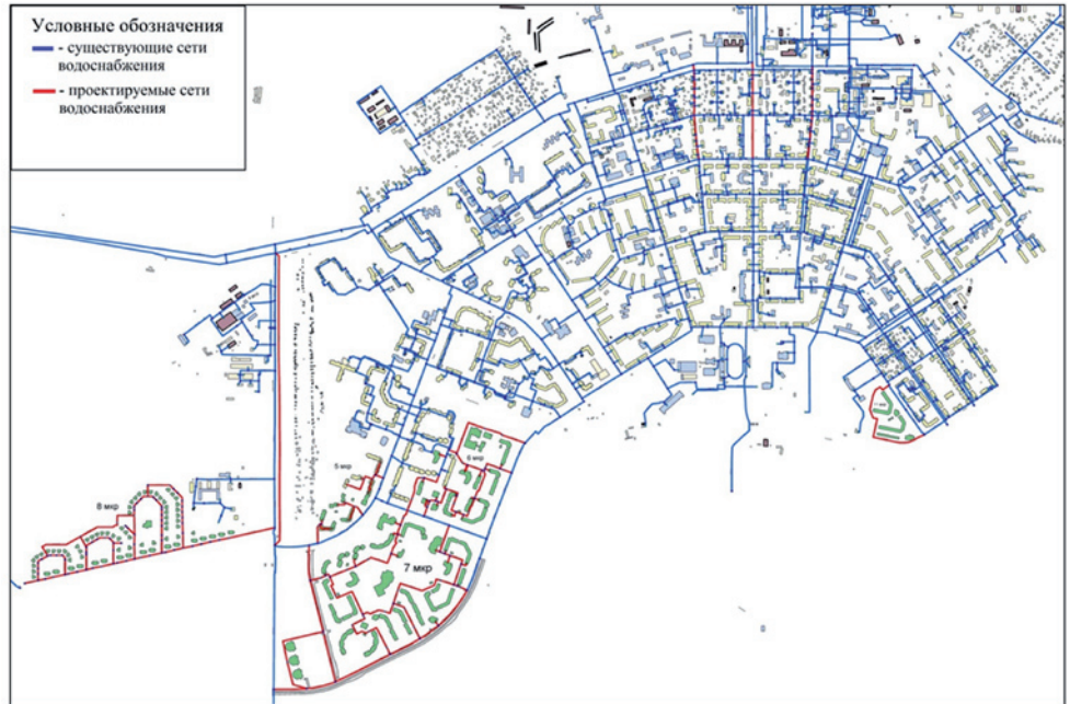
Рисунок 25. Схема существующего и планируемого размещения объектов водоснабжения города Лесной
