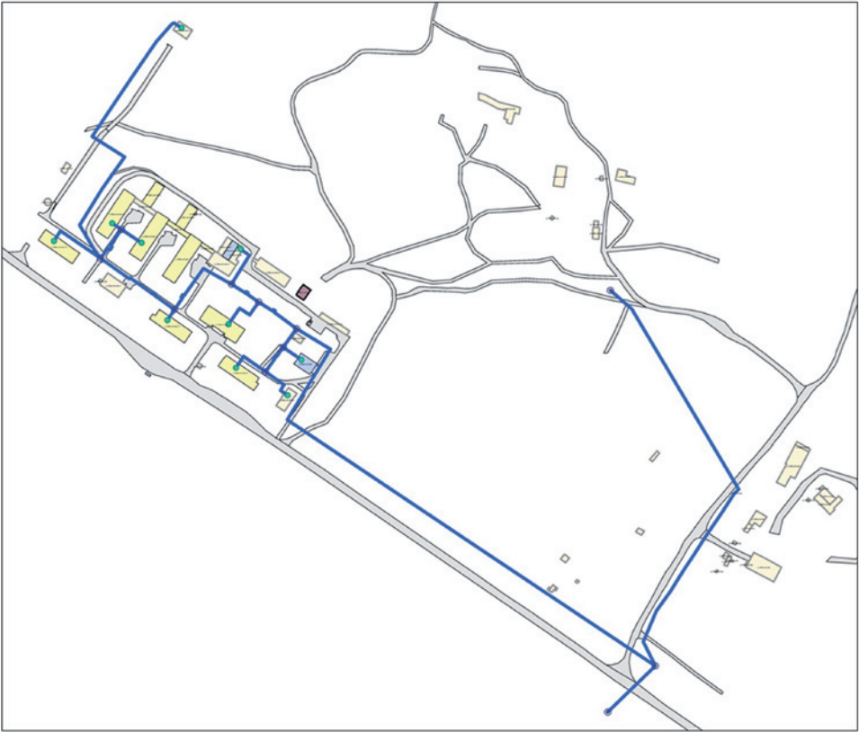
Рисунок 8. Схема расположения объектов системы водоснабжения р.пос. Ёлкино
