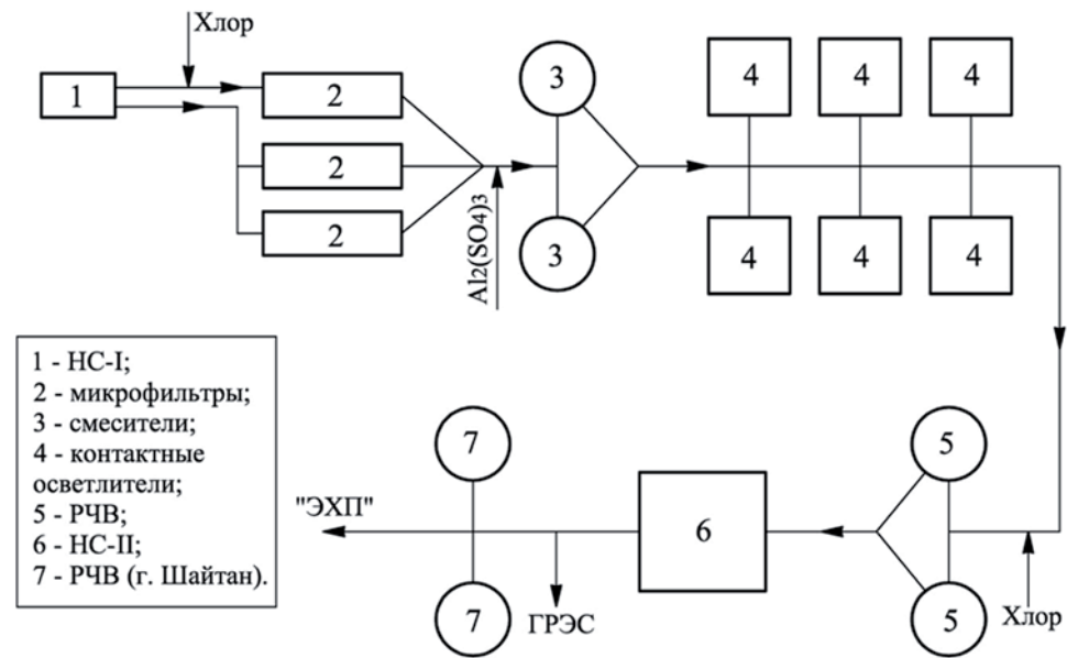
Рисунок 4. Технологическая схема забора и подготовки воды водозабора № 2
