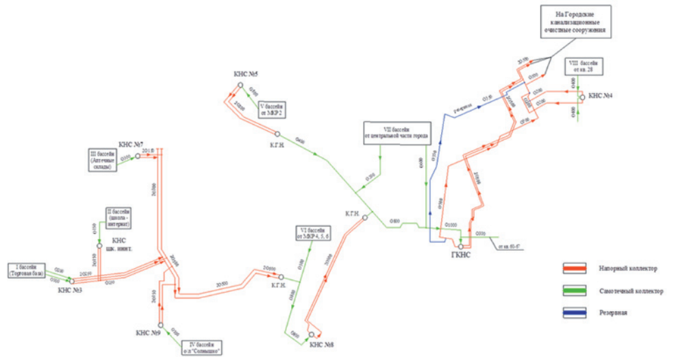
Рис. 2 Принципиальная схема передачи стоков по технологической зоне водоотведения города Лесной
