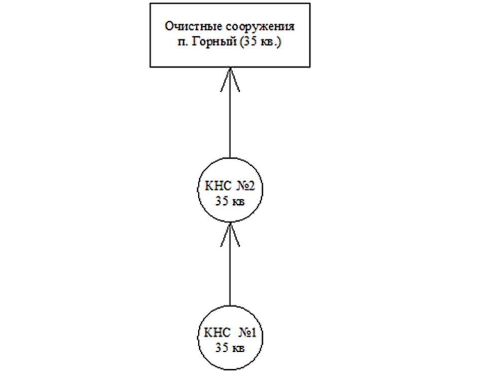
Рис. 6 Принципиальная схема передачи стоков по централизованной системе водоотведения 35 кв. г. Лесной
