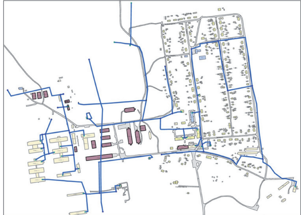
Рисунок 7. Схема расположения объектов системы водоснабжения пос. Чащавита
